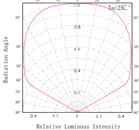
发光角度图
